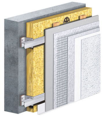
System H6-verputzt Hinterlüftete Fassade
