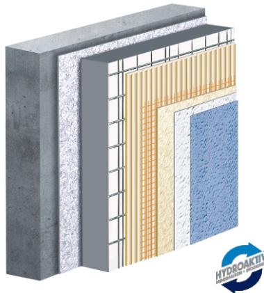
Kompaktsystem K5 AquaROYAL Polystyrol-Hartschaumplatte
