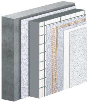
Kompaktsystem K5 EPS 030/031 grau Polystyrol-Hartschaumplatte
